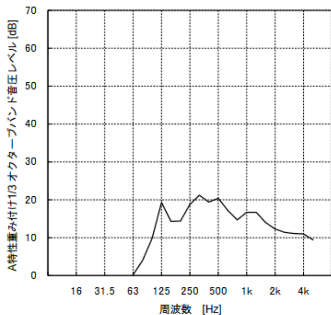
(a). 残留騒音の周波数特性
