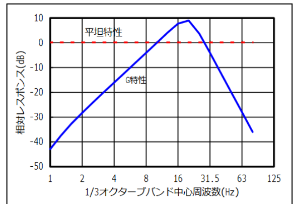
図-1.1 低周波音の周波数補正特性
