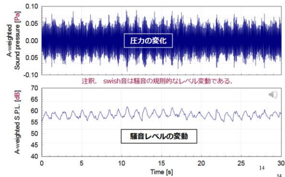
振幅変調音（AM変調音、swish音ともいう）
