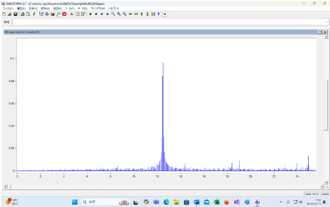
工場騒音 0～25Hz、最大音圧 0.1[Pa] （12.5Hz）
