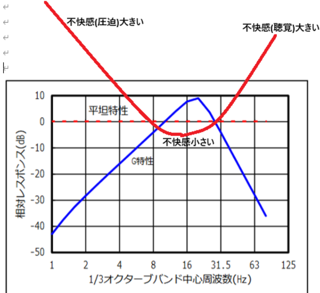
図-1.1 低周波音の周波数補正特性
