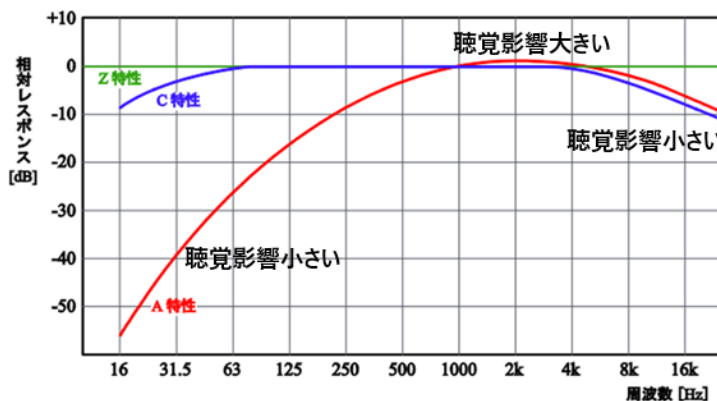
図2 周波数重み付け特性 A/C/Z
