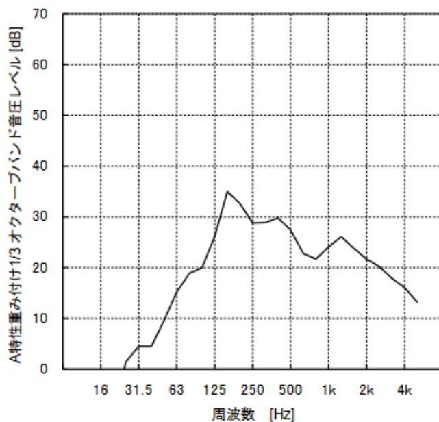
(b). 風車騒音の周波数特性
