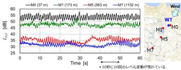
振幅変調音（騒音レベル L_{A,F} （A特性、Fast）の測定例）
