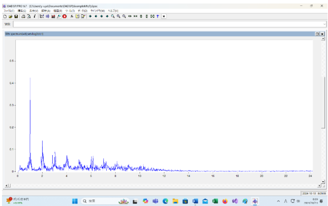
風車音（強風） 0～24Hz、最大音圧 0.42[Pa]（1Hz）
